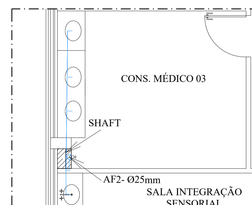
5 DETALHE 2 ESCALA : 1/50
