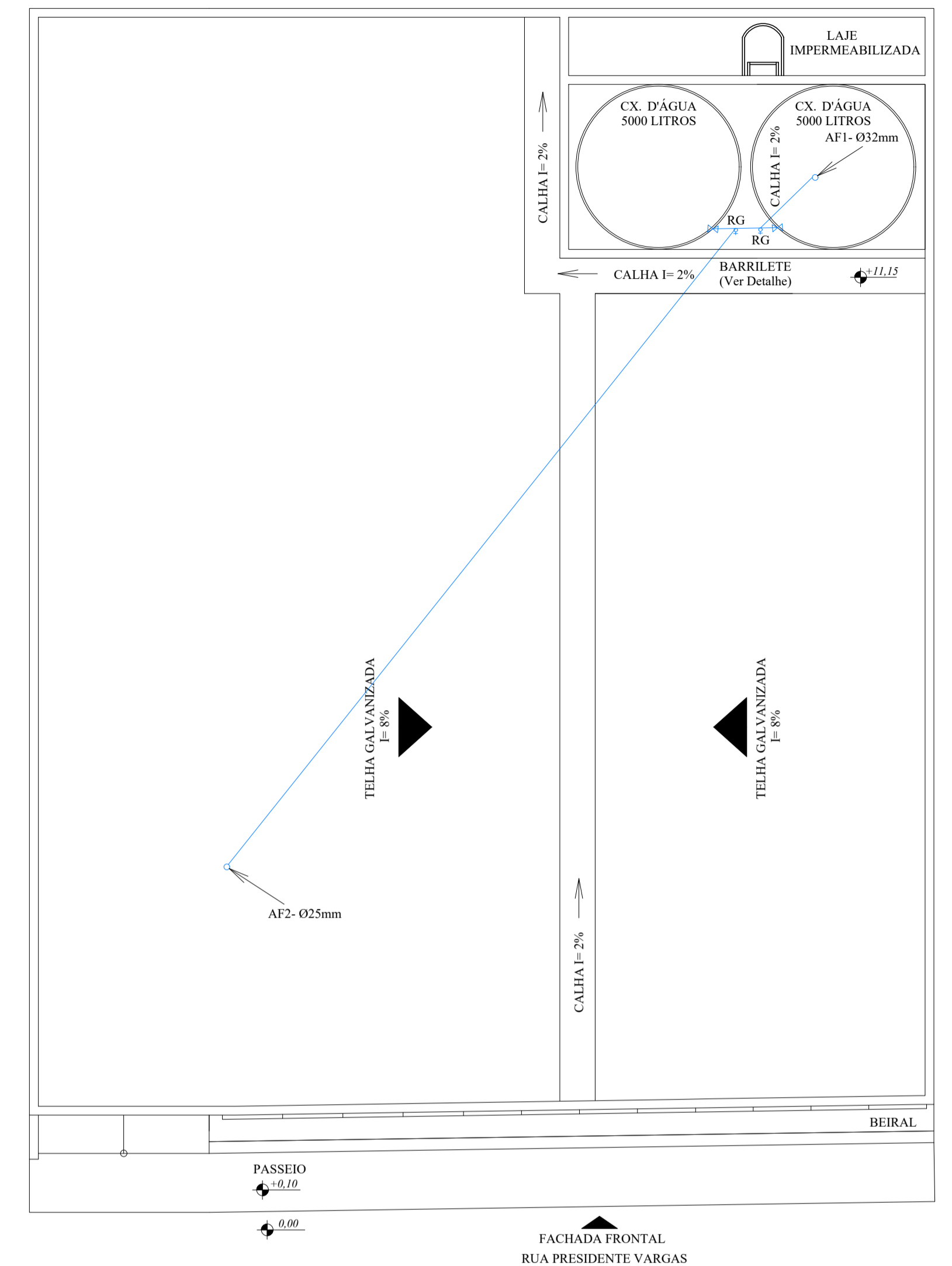
3 PLANTA BAIXA ÁGUA FRIA - COBERTURA ESCALA : 1/75
