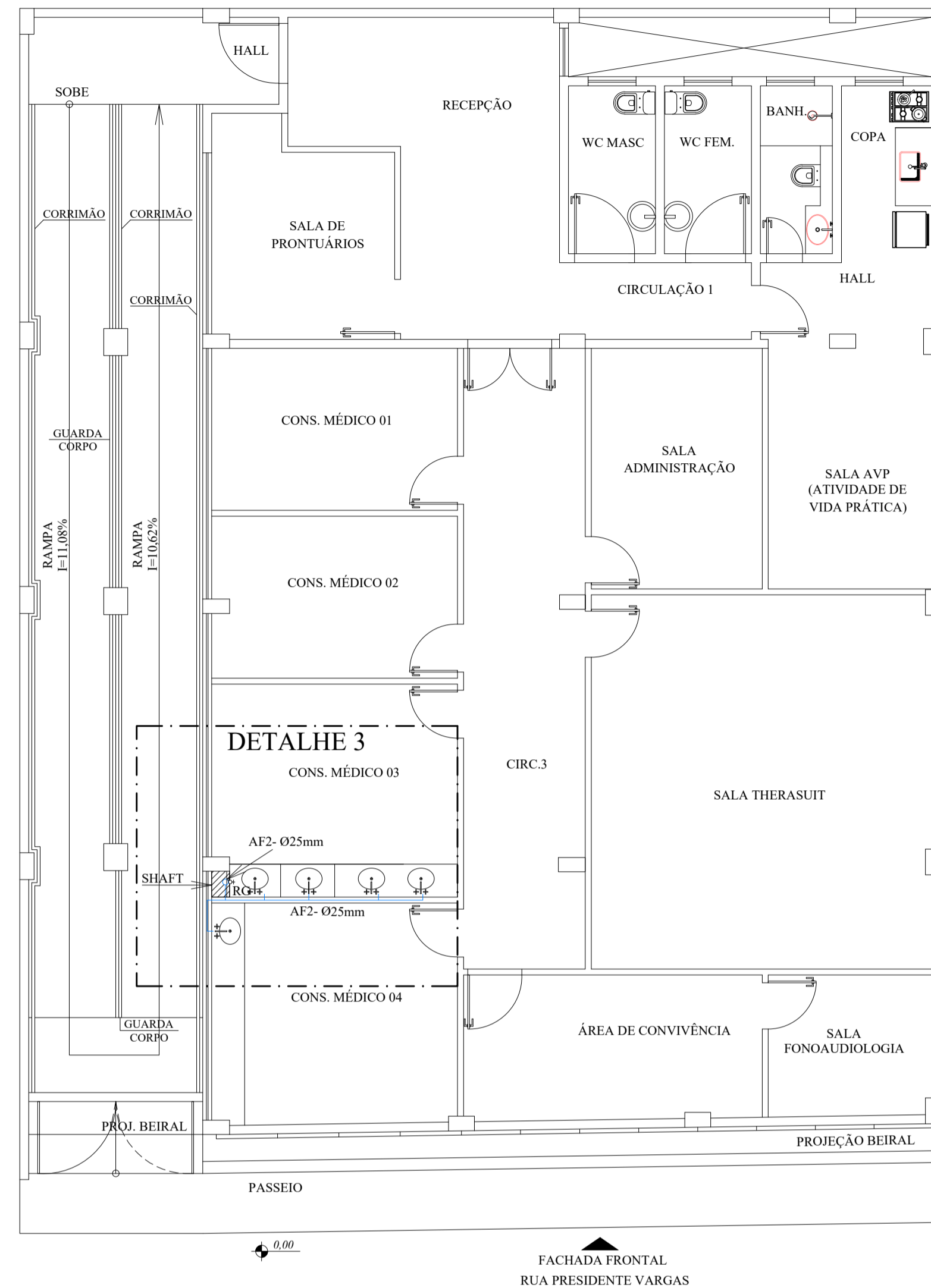
1 PLANTA BAIXA ÁGUA FRIA - 1º PAVIMENTO ESCALA : 1/100
