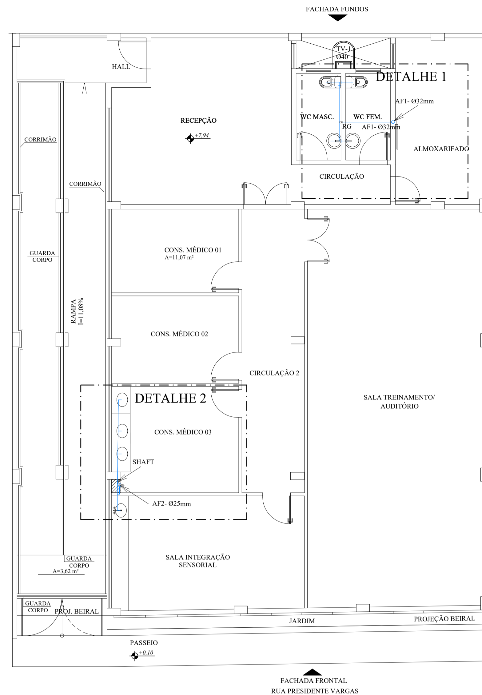
2 PLANTA BAIXA ÁGUA FRIA - 2º PAVIMENTO ESCALA : 1/75
