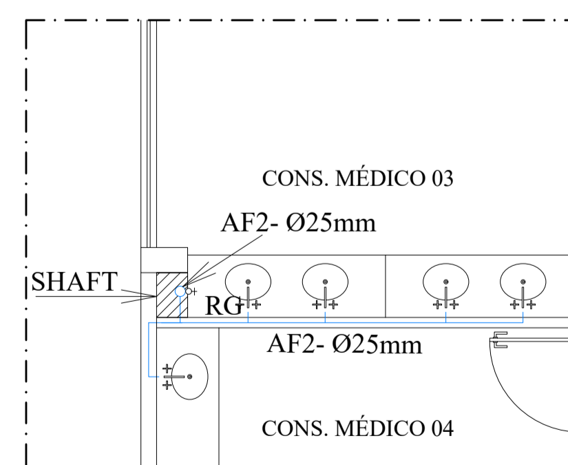
6 DETALHE 3 ESCALA : 1/50
