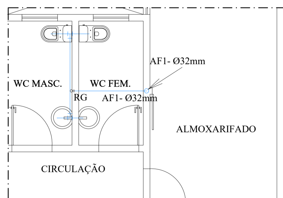
4 DETALHE 1 ESCALA : 1/50
